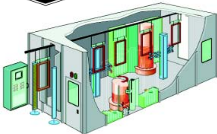
Kompletny system firmy Reiter: Automatyczna lakiernia okien Kontur V
